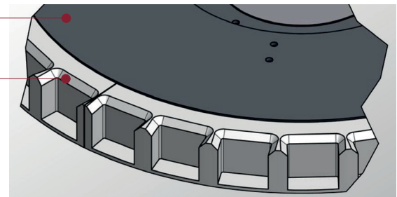
Selettore a più cavità (simulazione 3D)
