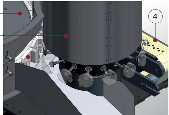
Interno del riordinatore POSIBOT (simulazione 3D)
