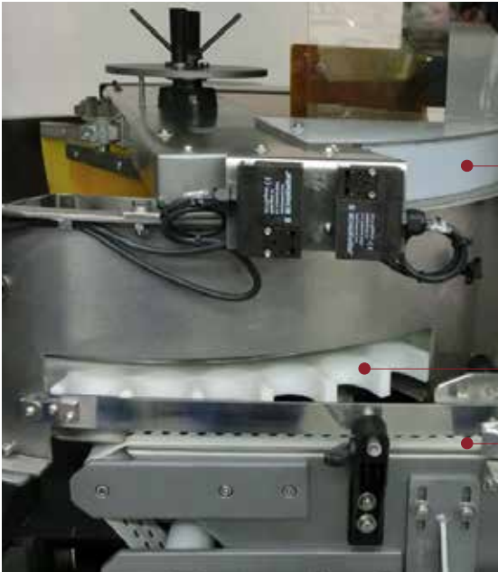
POSIPHARMA款-13型理瓶机内部
