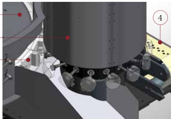
POSIBOT整理机内部 (3D模拟)
